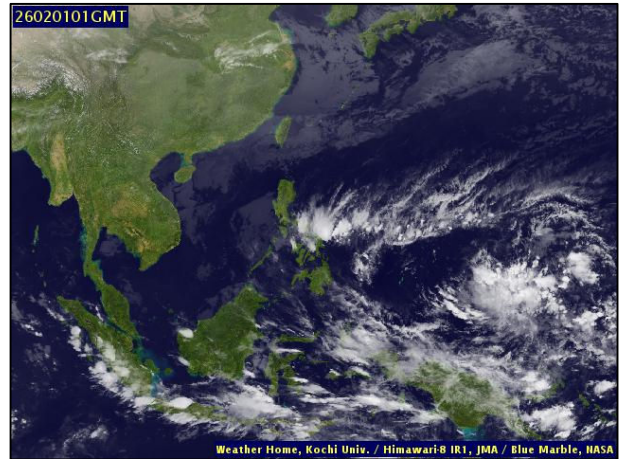
ภาพถ่ายดาวเทียม วันที่ ๑ ก.พ. ๒๕๖๙ เวลา ๐๘.๐๐ น.
